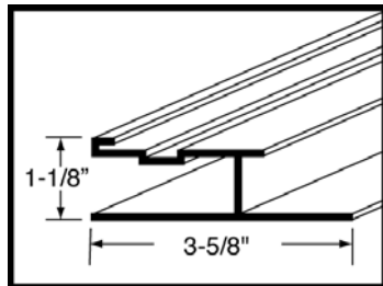
Inwall # 1 Gunite # 1040P
