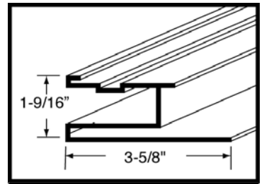
Inwall # 4 Fiberglass #1301P
